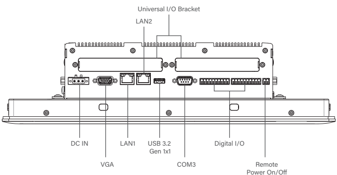
Right I/O
