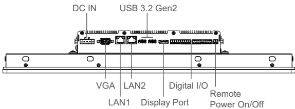
Right I/O
