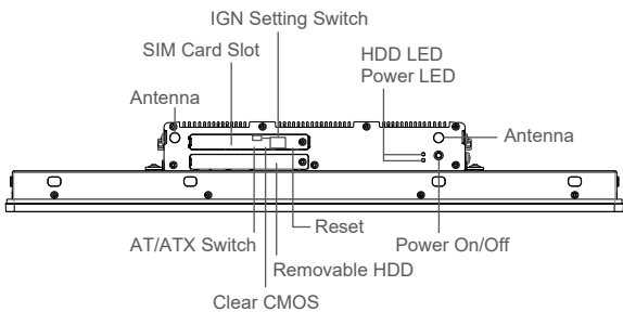
Left I/O
